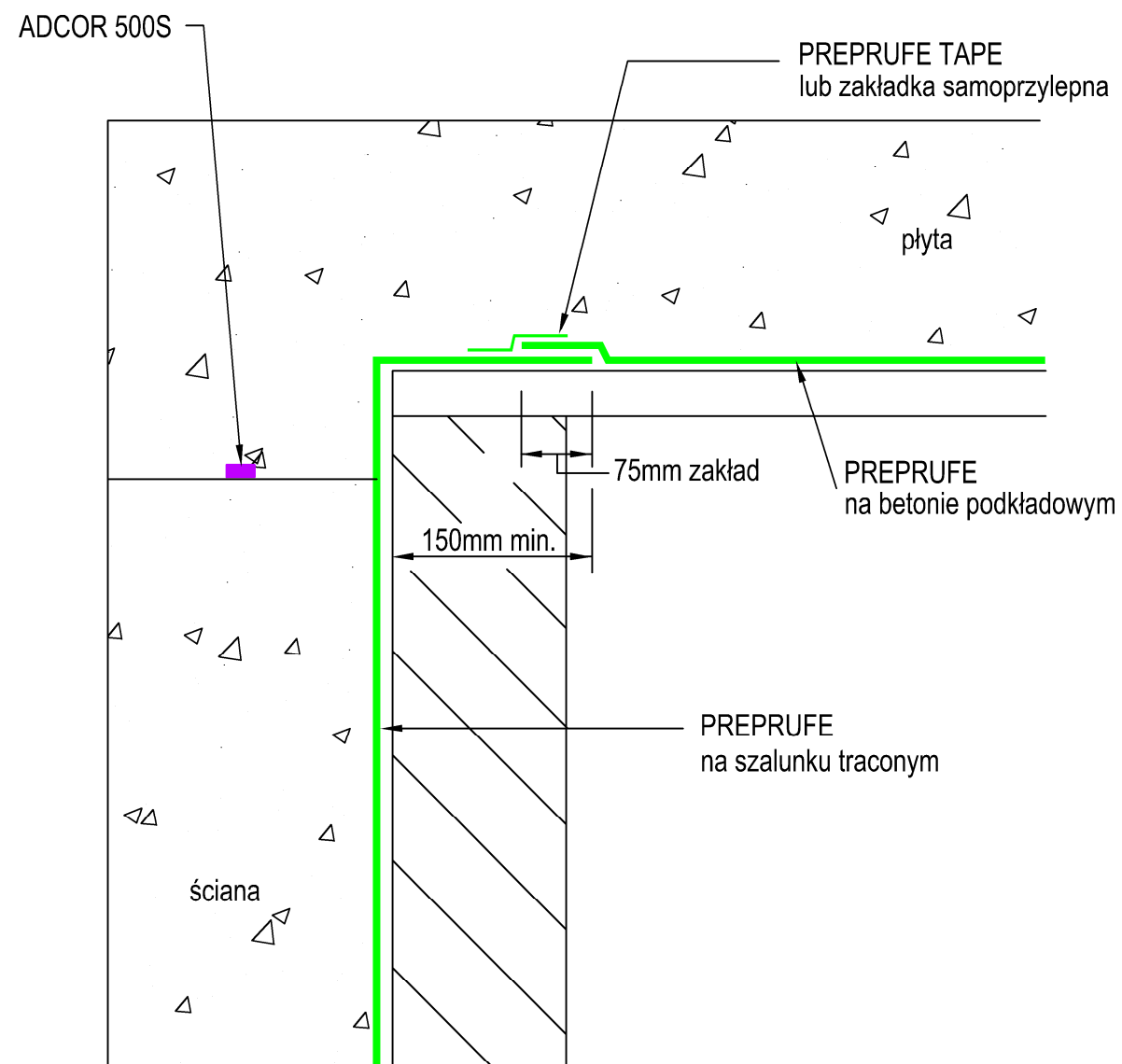
DETAL POŁĄCZENIA ŚCIANY I PŁYTY NA GRUNCIE PRZEKRÓJ
